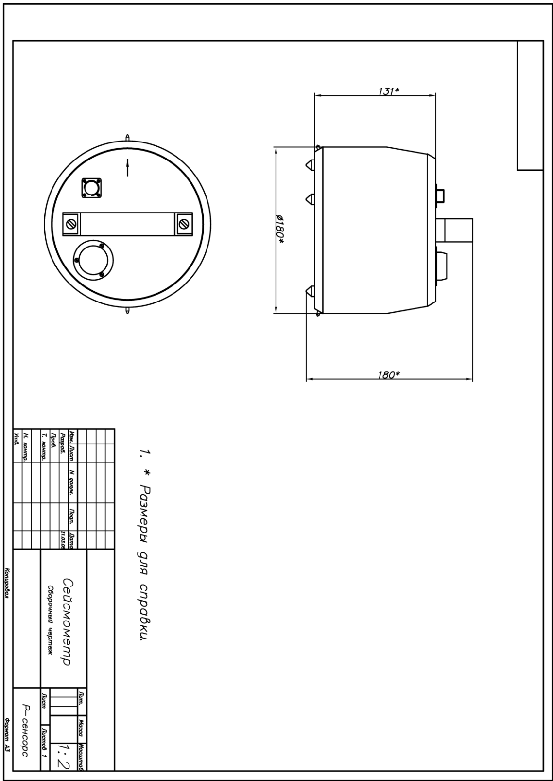
Рис. 3. Габаритный чертеж сейсмометра СМЕ-4311.
