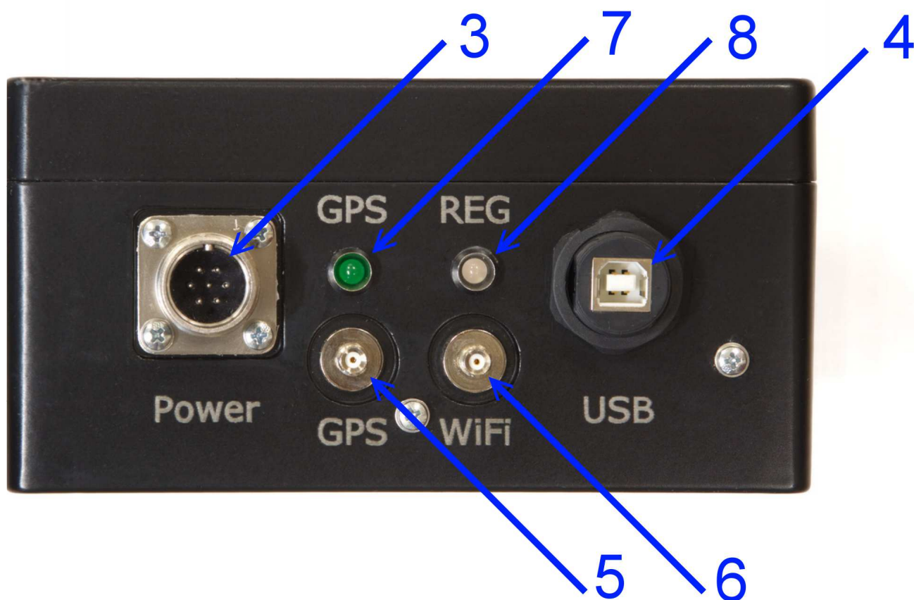
Рис. 2. Разъемы и светодиоды
