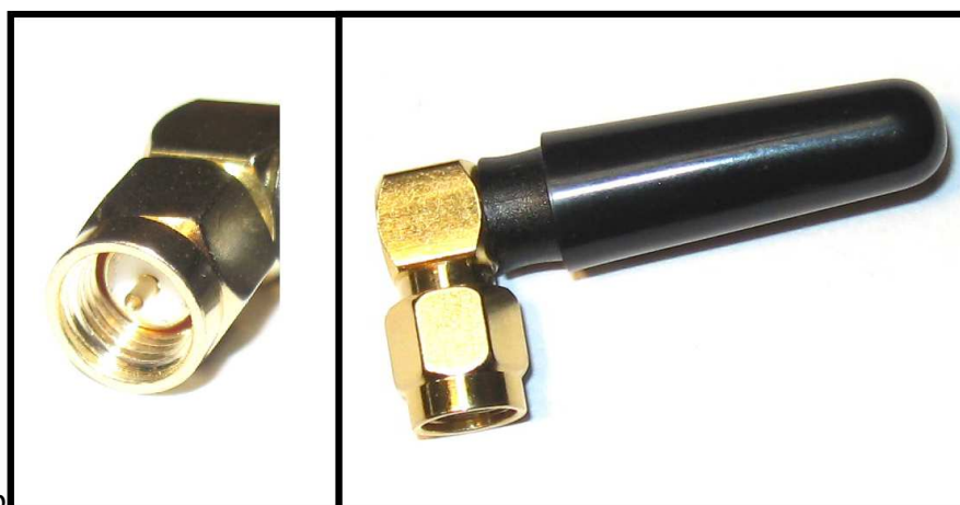
Рис. 7. Антенна WiFi – разъем, внешний вид (внешний вид антенны в комплекте поставки может отличаться от представленного)
