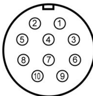
2PM(Г)22Б10Ш1Е2 male connector 2PM(Г)22Б10Ш1Е2 вилка
