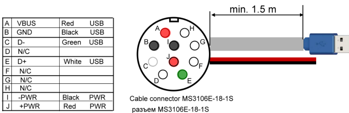
Рис. 1. Многофункциональный разъем, комбинированный кабель.
