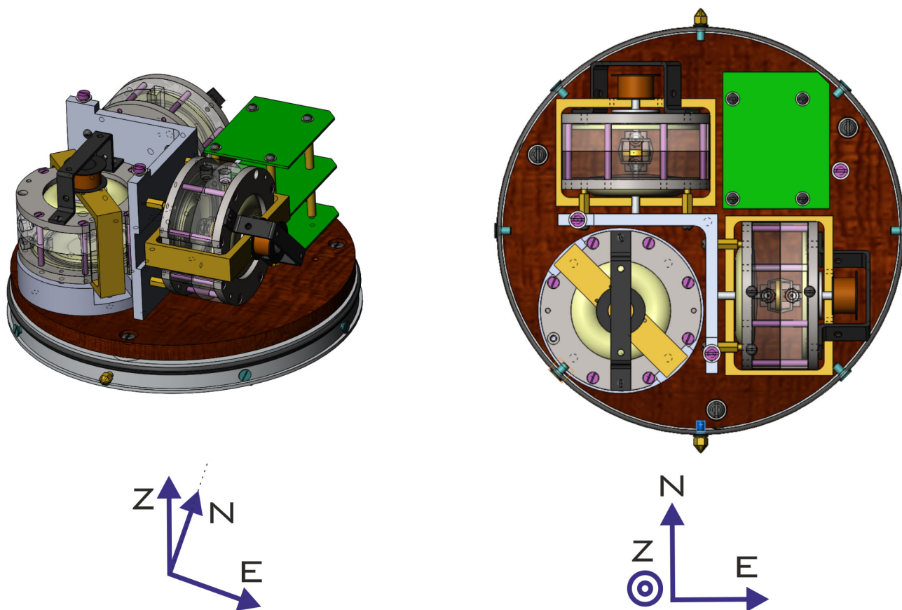
Рис.1 Геометрия чувствительных элементов сейсмометра СМЕ-6011ND.
