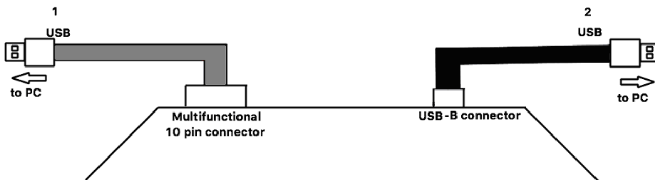
Рис. 11 Подача питания от USB для цифровой подсистемы
