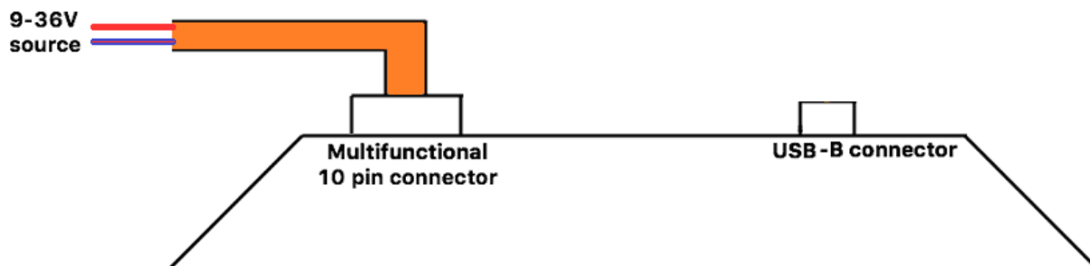
Рис. 10 Подача питания по кабелю питания (основной режим работы)
