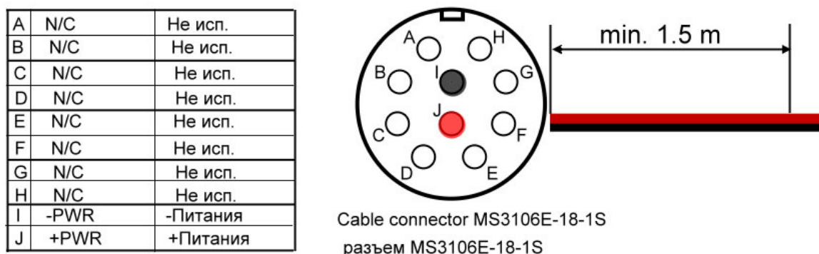
Рис. 2. Многофункциональный разъем, Кабель питания
