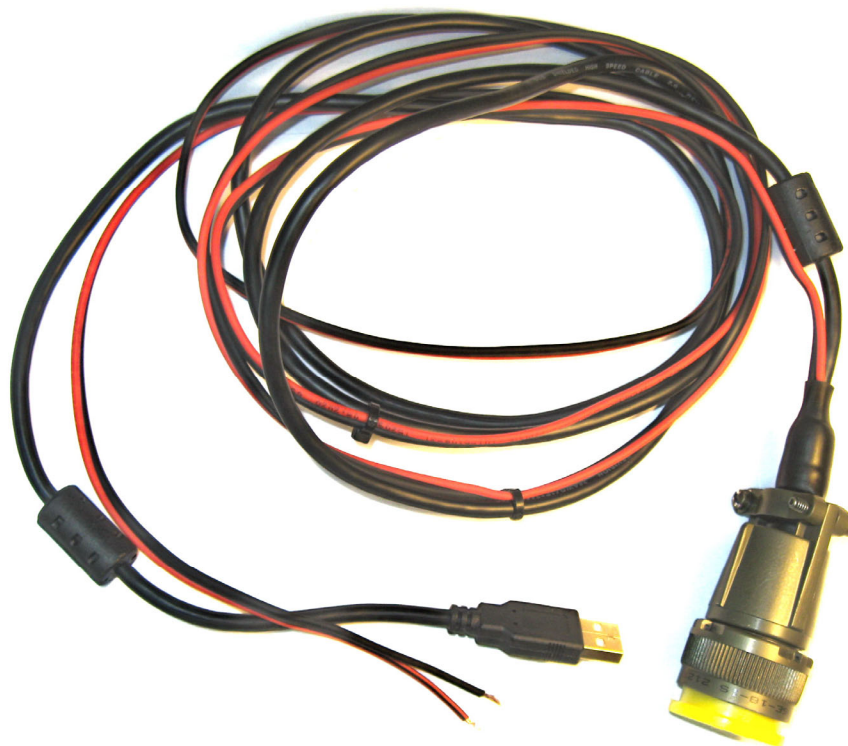
Рис. 3. Комбинированный кабель.
