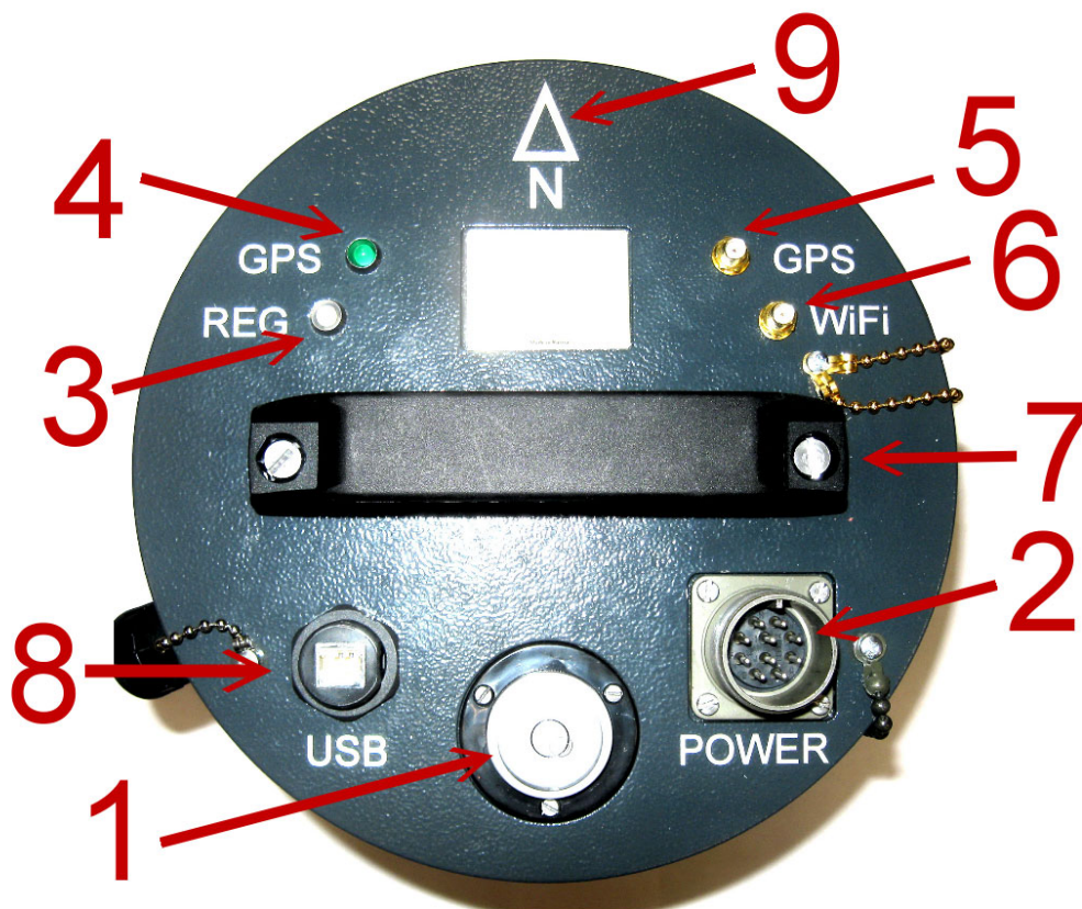
Рис. 1. Разъемы и индикаторы
