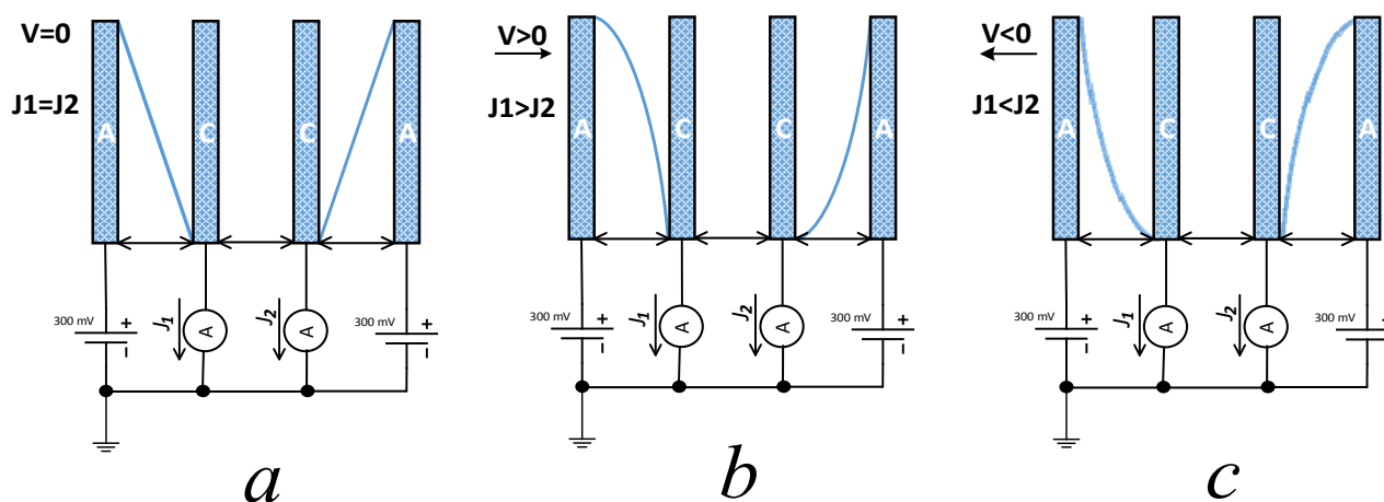
Рисунок 2. Распределение концентрации активного компонента в растворе электролита. (а – состояние покоя, б и с – движение вправо и влево соответственно).
