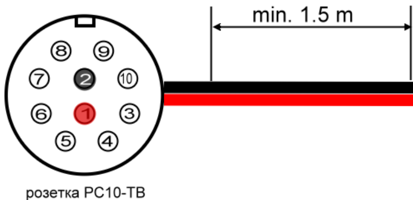
Рис. 2. Многофункциональный разъем, Кабель питания
