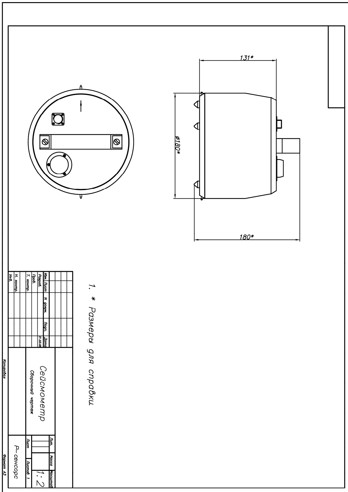
Рис. 3. Габаритный чертёж сейсмометра СМЕ-4211.
