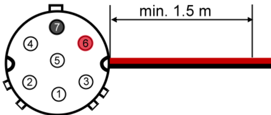
DH-20-J07PE-03-001A розетка
